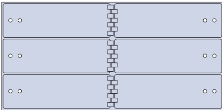
TLX-6 (Wt. 190 lbs.) 6 openings ea. 4 1/2" x 15"
